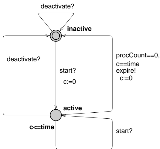
Fig. 10. The Timer automaton.
