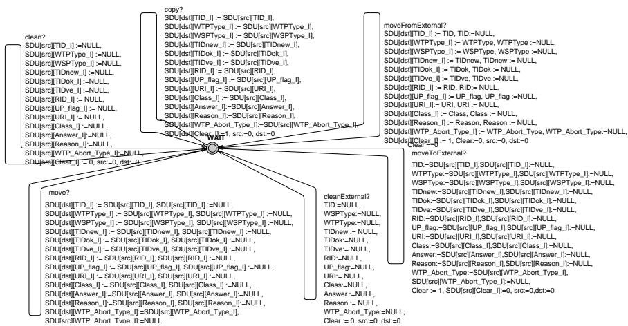
Fig. 9. The Datstore automaton.
