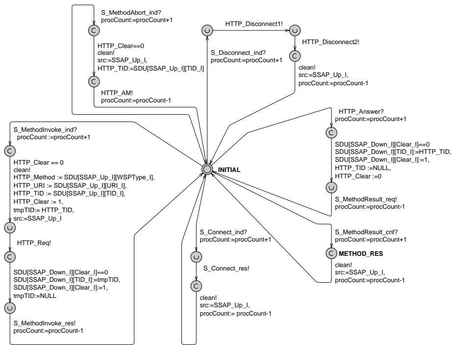
Fig. 14. The SSAP automaton.
