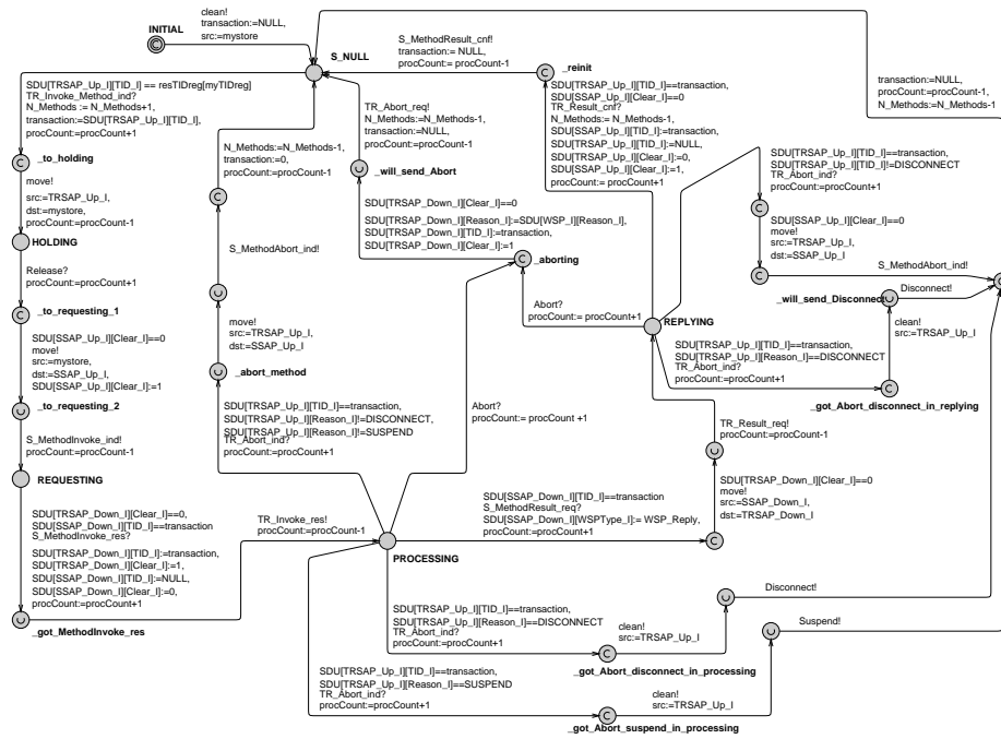
Fig. 13. The Method automaton.
