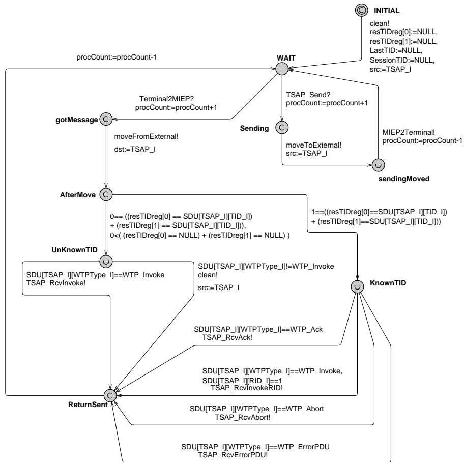
Fig. 8. The TSAP automaton.
