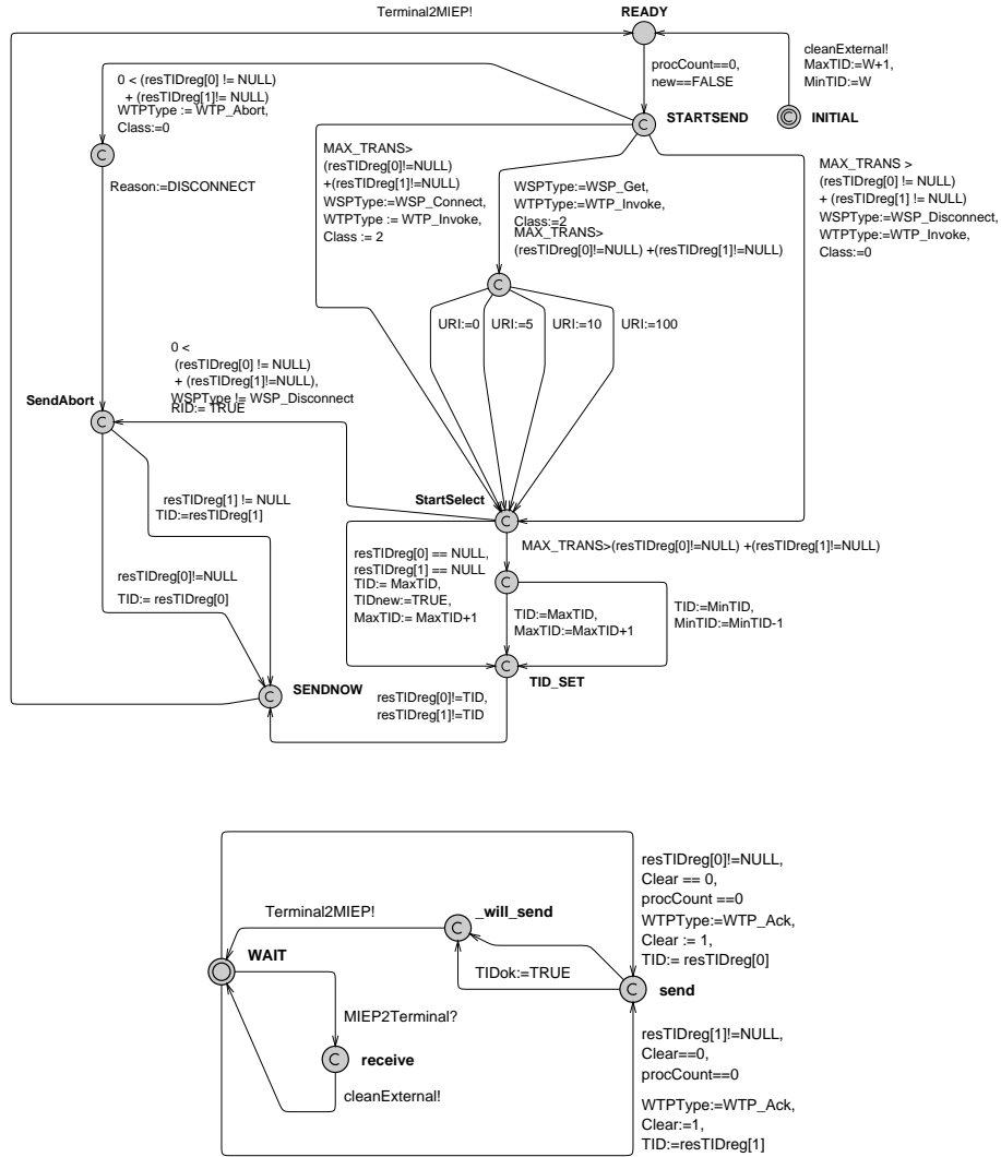
Fig. 7. The Terminal automata.
